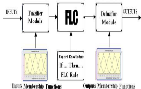
Fig.8. Fuzzy Basic Module
