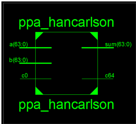
Fig. 2: RTL SCHEMATIC
