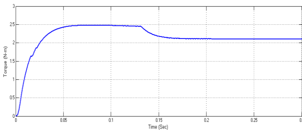
Fig.11 Torque.
